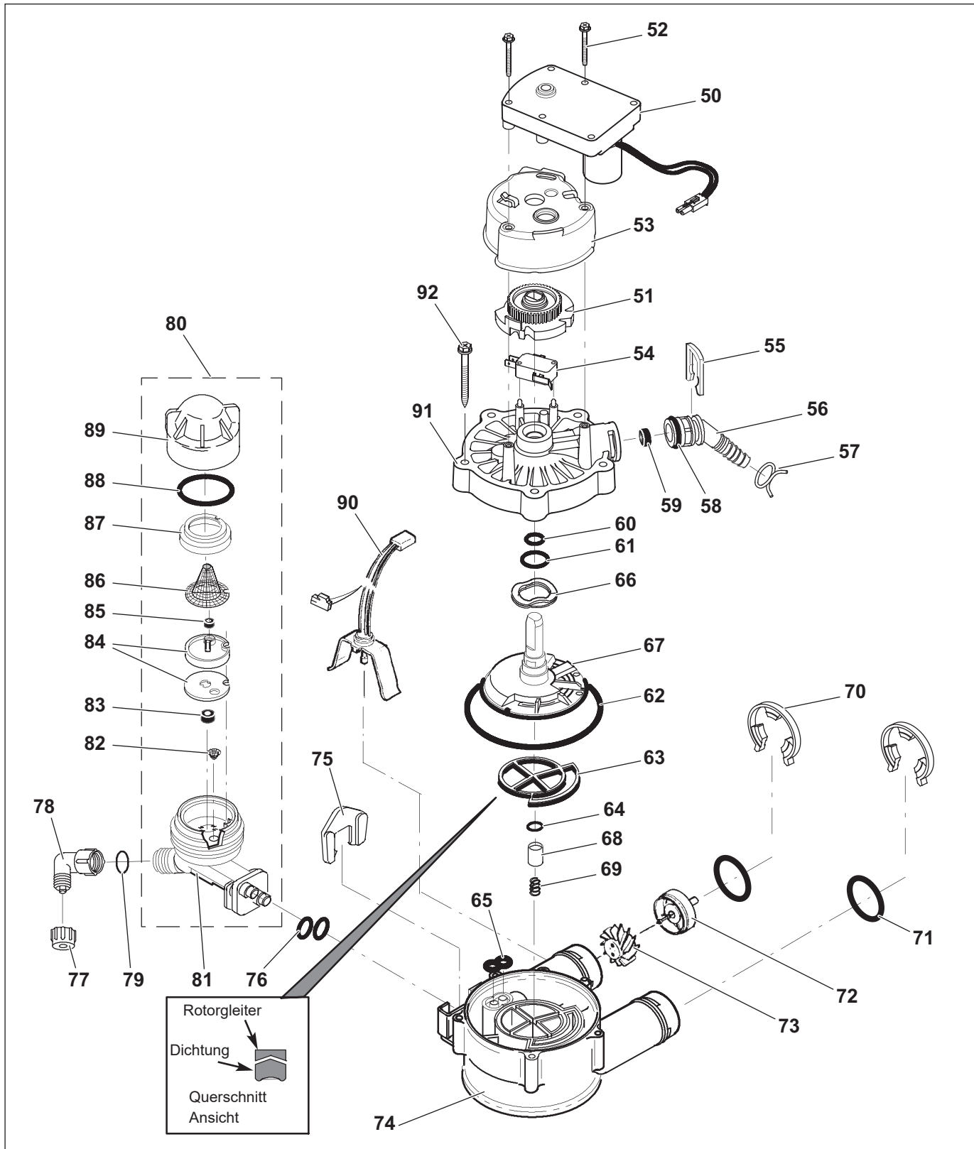
Abb. 19: Ventilbaugruppe
