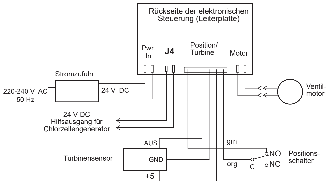
Abb. 22: Leiterplatte
