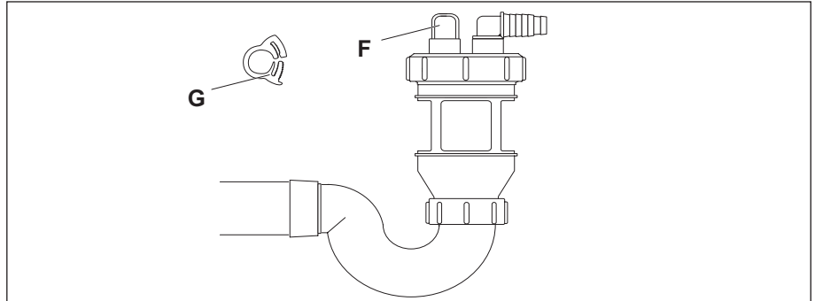
Abb. 8: Abwasseranschluss
