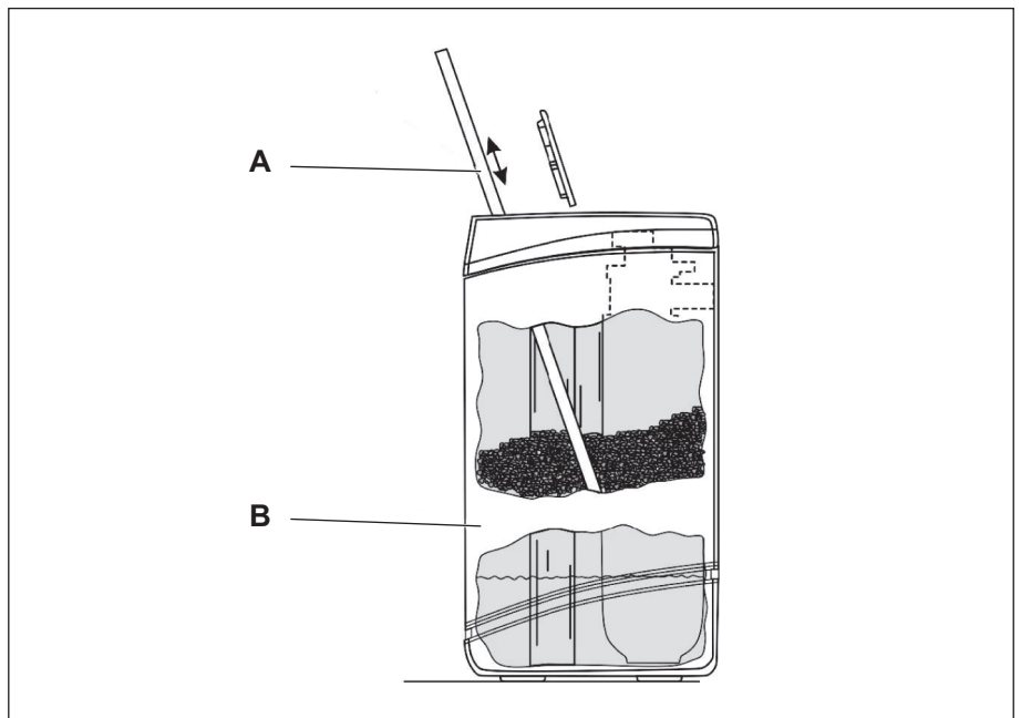
Abb. 17: Salzbrücke aufbrechen
