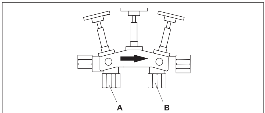
Abb. 12: Verschneidearmatur
