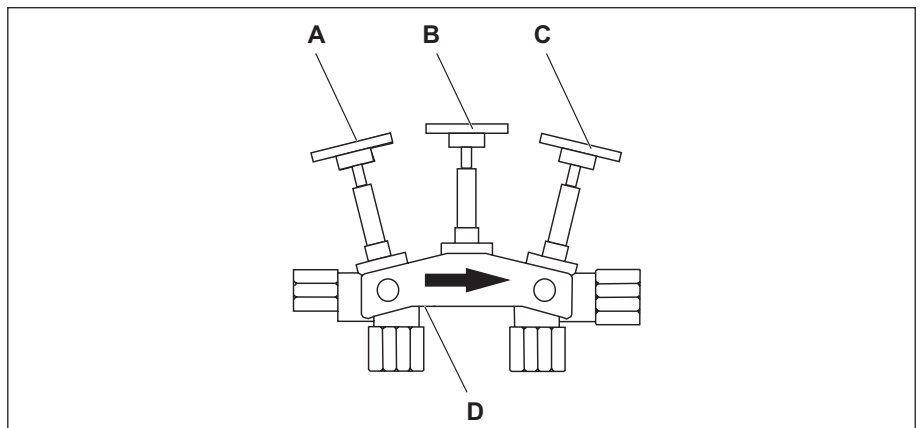
Abb. 14: Verschneidearmatur
