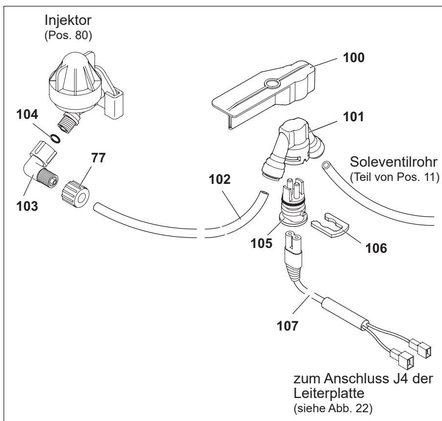
Abb. 20: Chlordesinfektionseinheit
